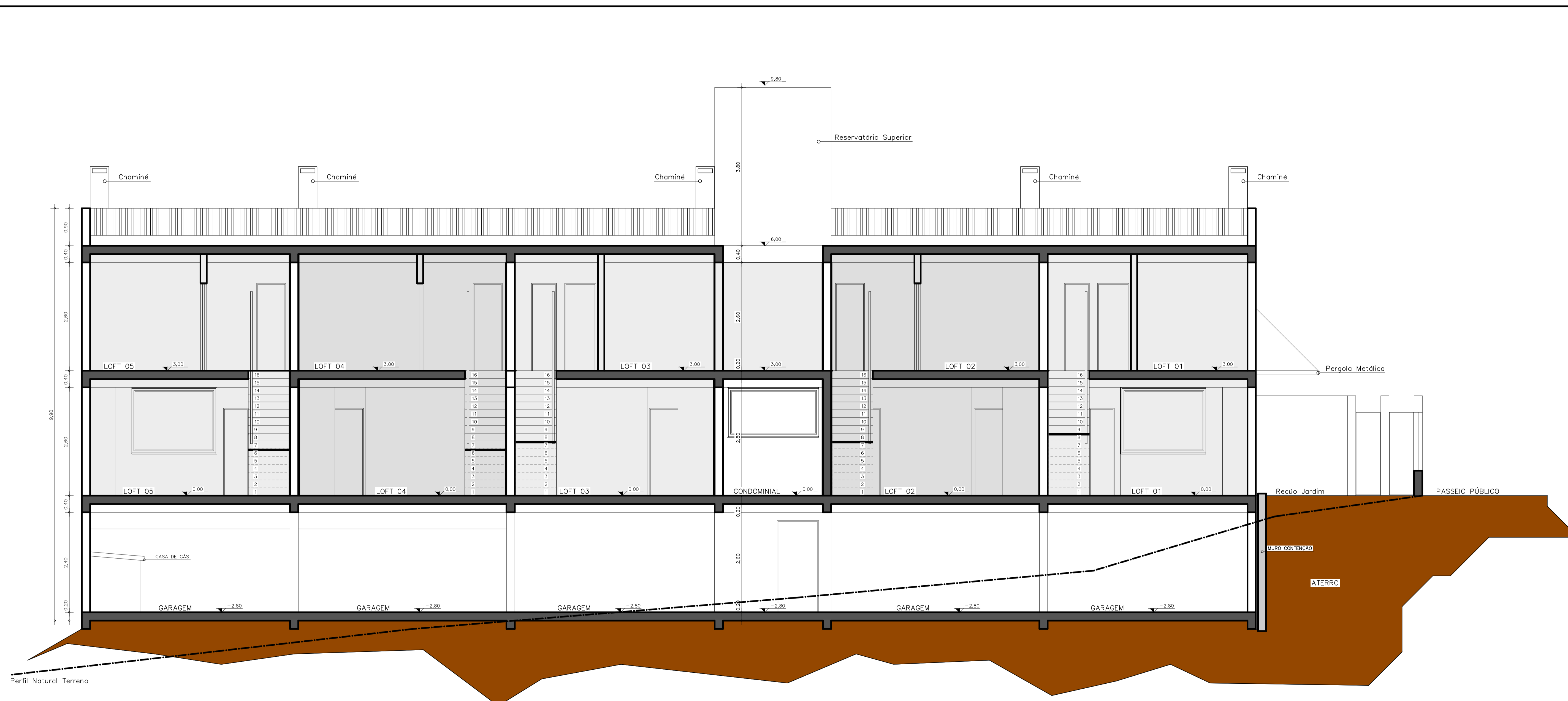
CORTE AA
